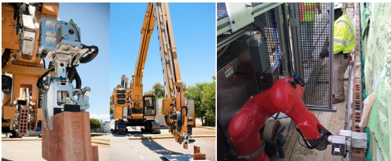
Εικόνα 2: Αριστερά: Fastbrick Robotics Hadrian και δεξιά: Construction Robotics SAM
