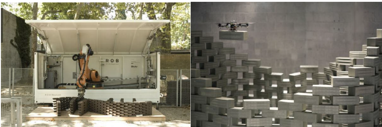
Εικόνα 1: Ρομποτικές διατάξεις χτισίματος τούβλων
