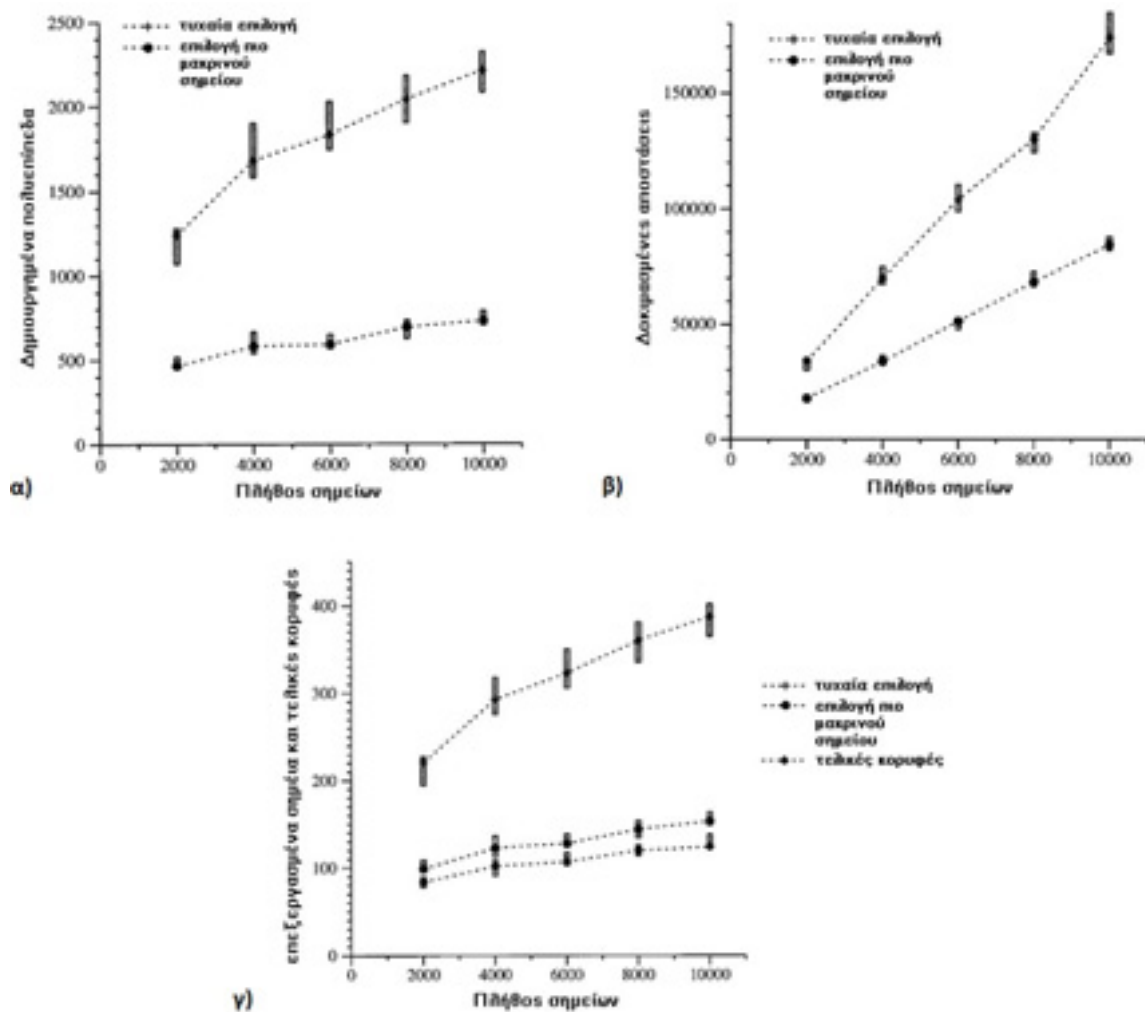
Σχήμα 1: Κυρτό περίβλημα ομοιομόρφως κατανεμημένων τριδιάστατων σημείων. Κατά μέσο όρο 10 δοκιμές για (α) δημιουργία πολυεπιπέδων, (β) δοκιμασμένες αποστάσεις, (γ) επεξεργασμένα σημεία και κορυφές στην έξοδο.
