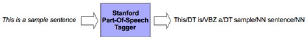
Σχήμα 3: POS-Tagging
