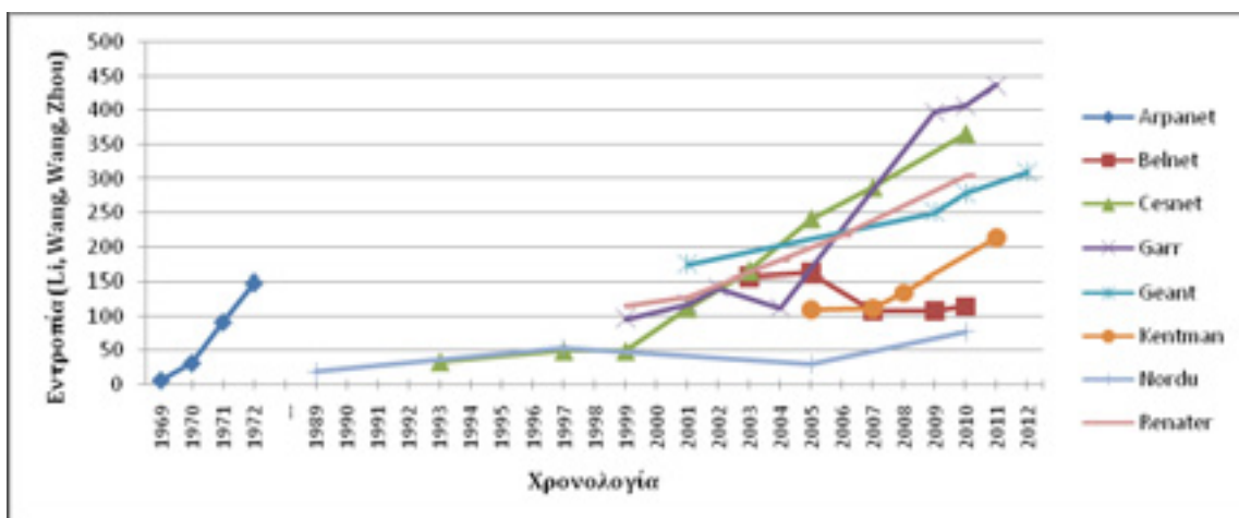
Σχήμα 7: Συγκεντρωτικό γράφημα εξέλιξης της εντροπίας με βάση Li, Wang, Wang, Zhou [11]
