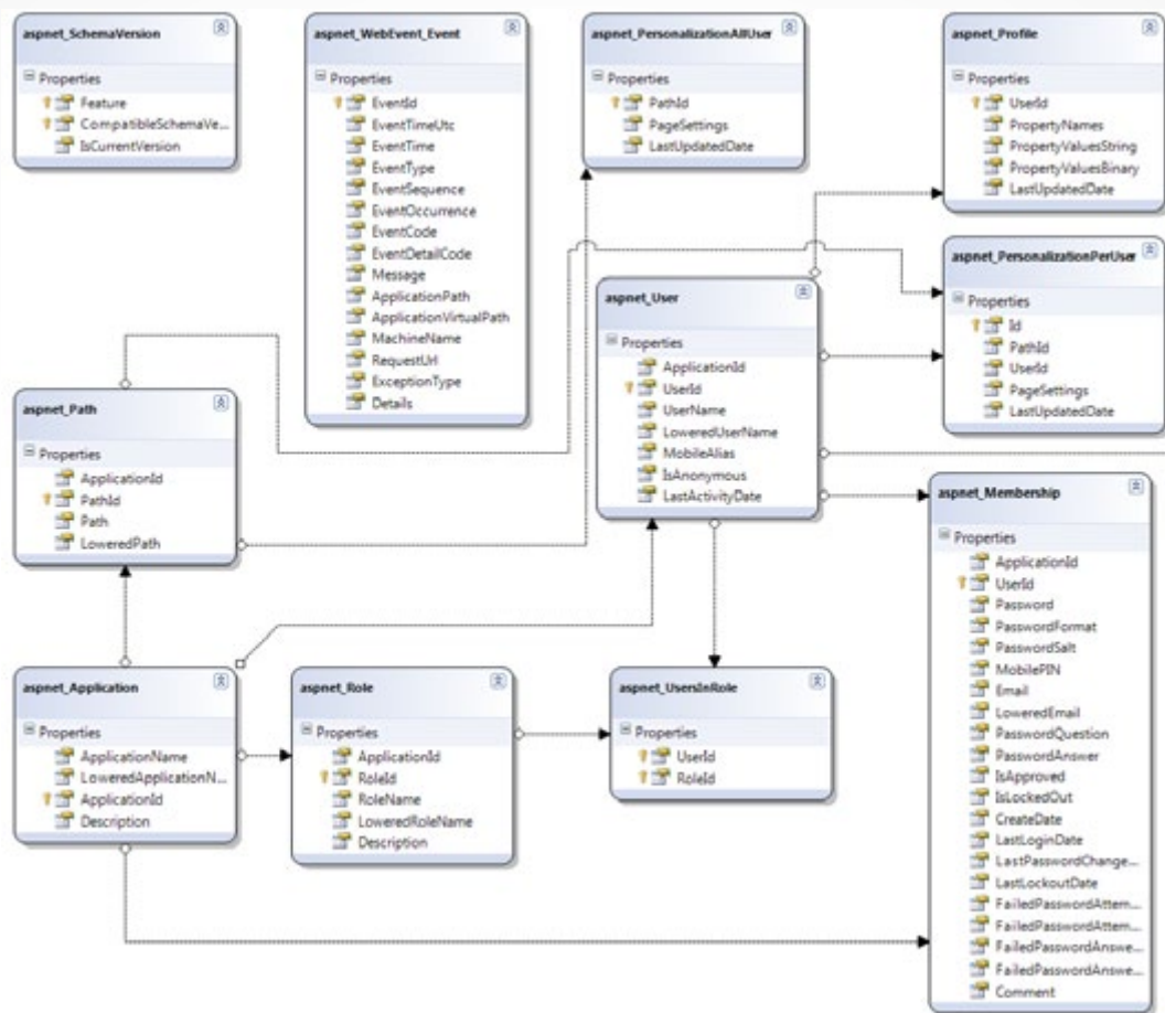
Σχήμα 2: Σχεδιασμός Βάσης Δεδομένων Συστήματος
